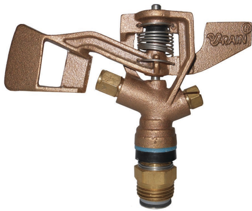
1/2" Dual Nozzle 23°x 7° 50-WSL
